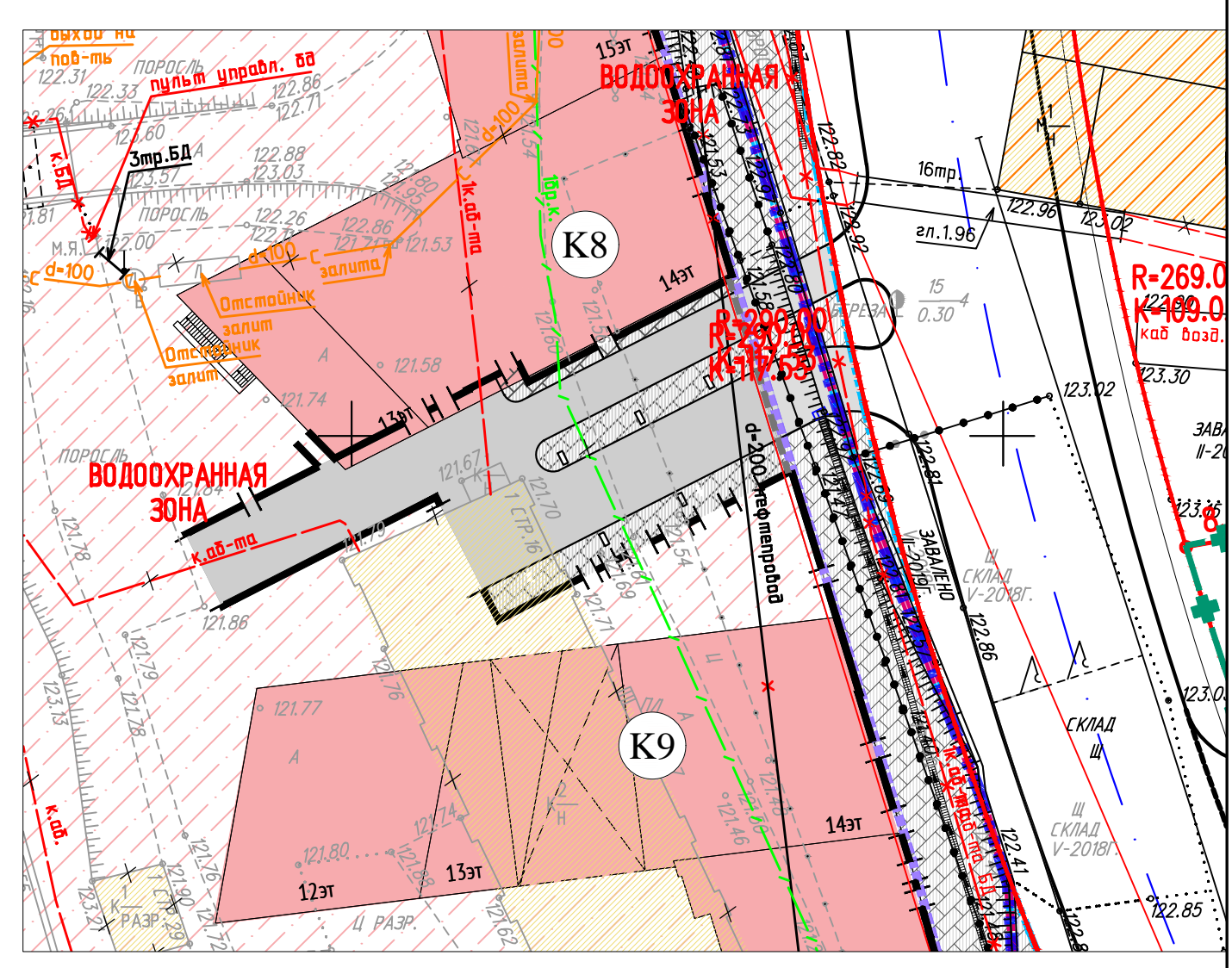
ФРАГМЕНТ 1. План на уровне 1 этажа М 1:500
